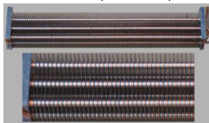
EVAP ESTAT BATEA 6 TUBOS 1700MM (CAÑO 1/2)
