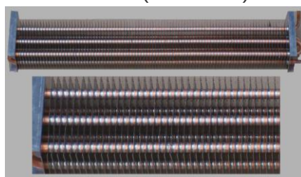
EVAP ESTAT BATEA 8 TUBOS 2100MM (CAÑO 1/2)
